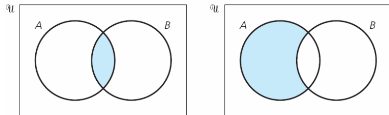
(c) A \cap B (d) A - B 37
