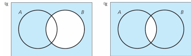
(c) \bar{B} (d) \overline{A \cap B} 38
