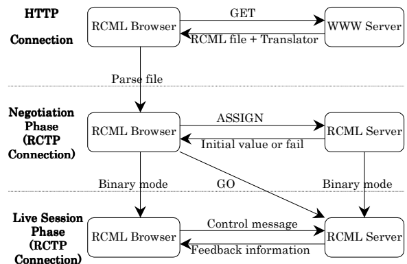
図 4 RCML システムにおける制御実行のシナリオ Fig. 4 Scenario of one controlling session
